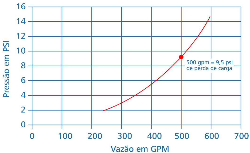
Gráfico de perda de carga
